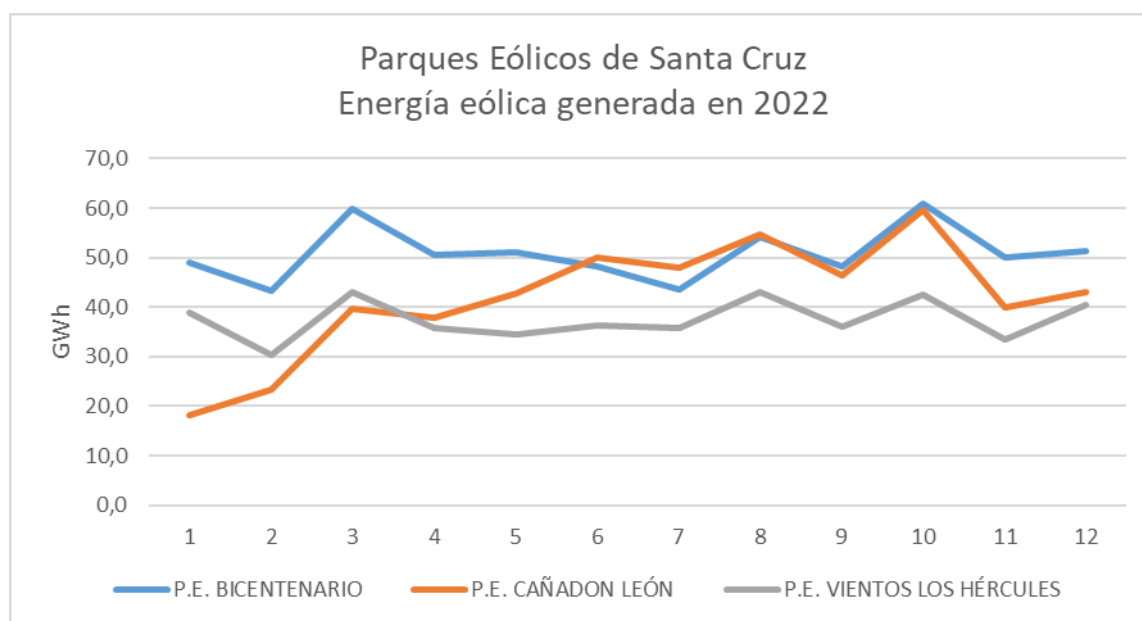
Figura 51 Producción mensual de energía eólica en 2022 en Santa Cruz (elaboración propia en base a [CAMMESA-ER,2022])
