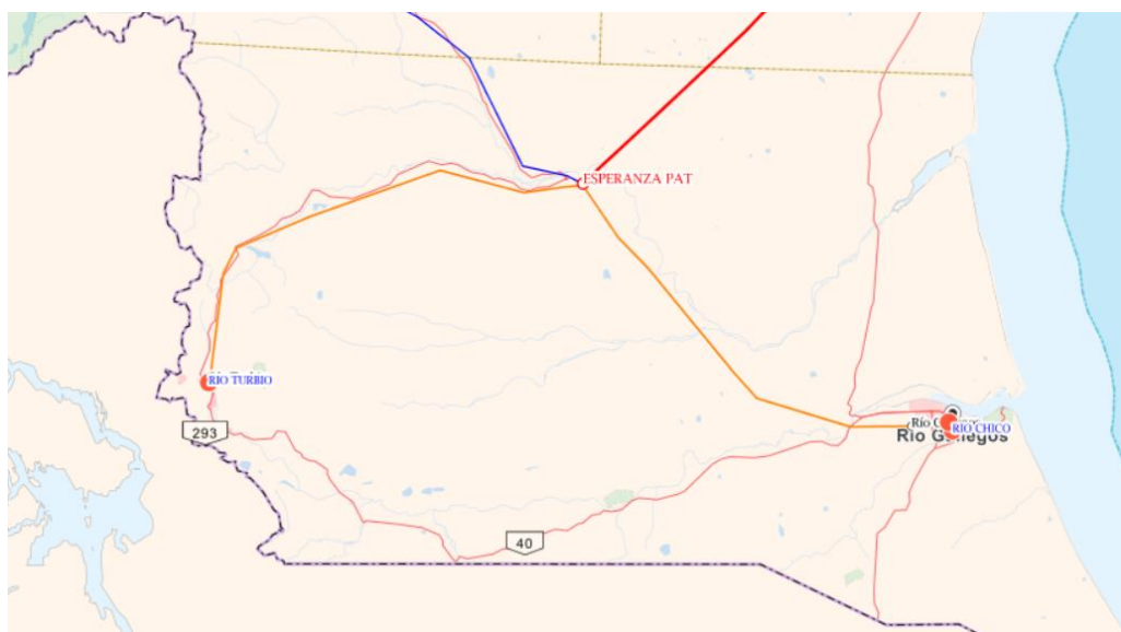
Figura 59 ubicación de la Central Río Turbio sobre línea 220 kV en el extremo sur del SADI [GEOSADI,2023]
