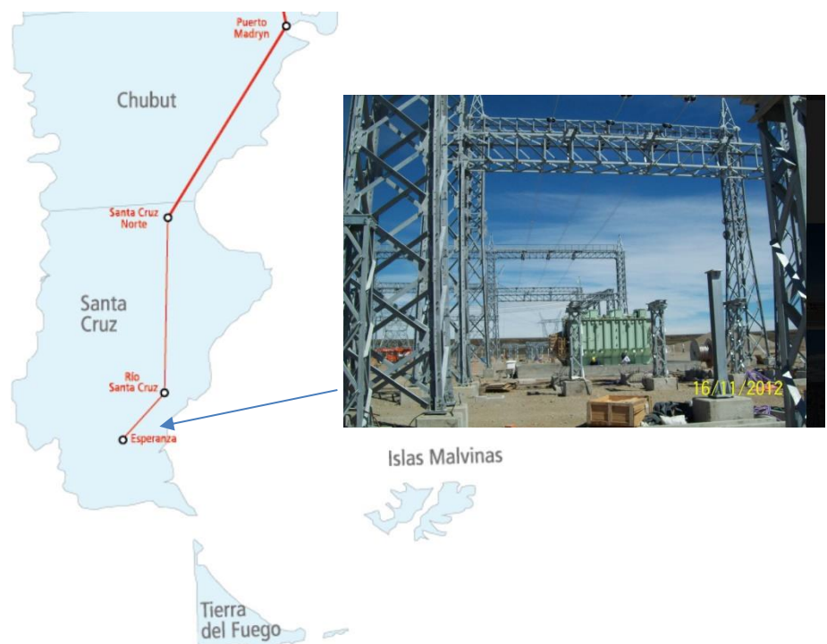
Figura 48 de la red de EAT (500 kV) del SADI hasta Pico Truncado/Santa Cruz Norte en 2008 y posteriormente en 2013 hasta Esperanza [Transener, 2022]
