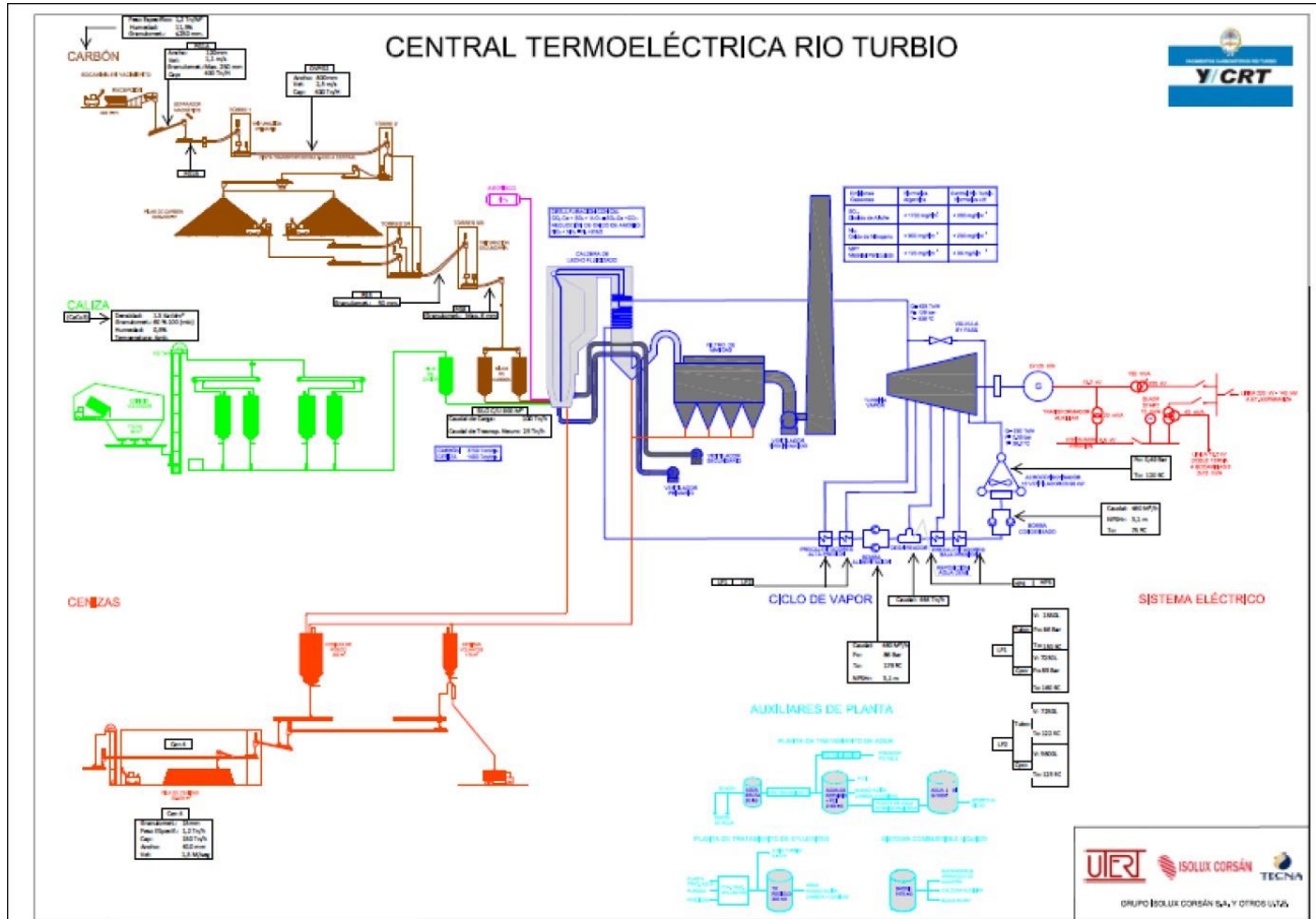
Figura 61 Diagrama de procesos CTRT [YCRT,2023]
