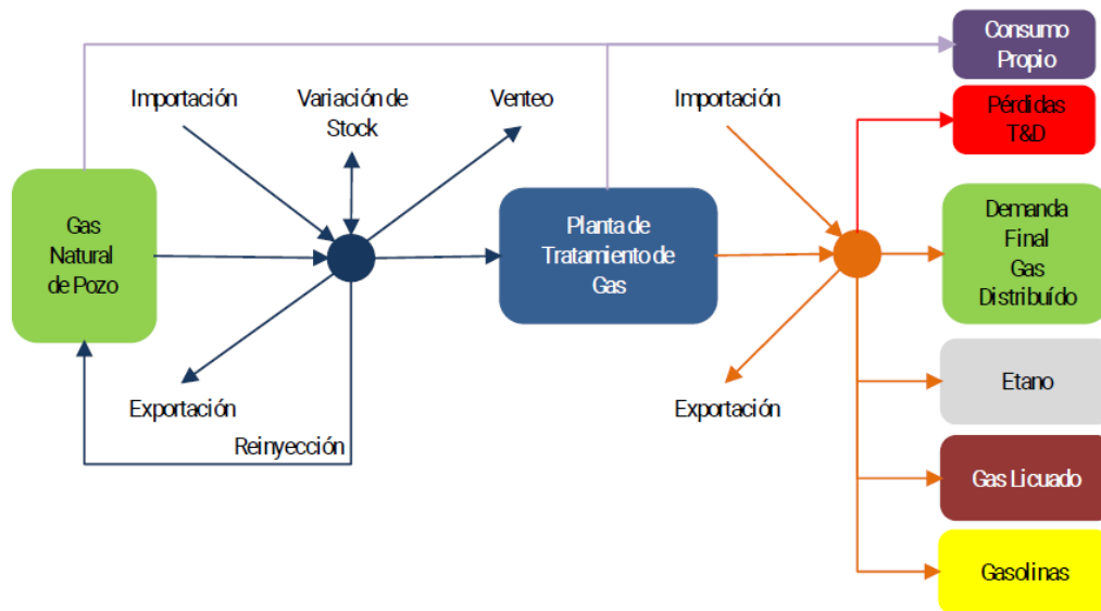
Figura 15 - Esquema de la cadena del gas natural según [MetodologíaBEN, 2015]
