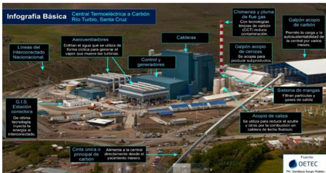
Figura 60 - Distribución de componentes en la CRTT [OETEC,2015]
