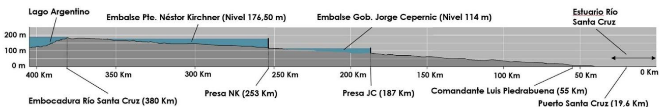
Figura 56 Distribución y cotas de las presas NK y JC [UNLP-RepresasSC,2017]
