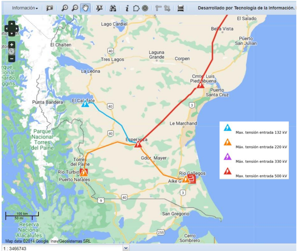
Figura 50 Vinculaciones al SADI en zona S y SW de Santa Cruz [SIG-ENERGIA, 2023]
