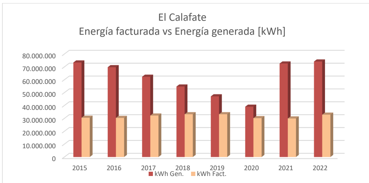
Figura 68 Comparativos entre energías facturada y generada / adquirida a SADI, para El Calafate (el.prop)
