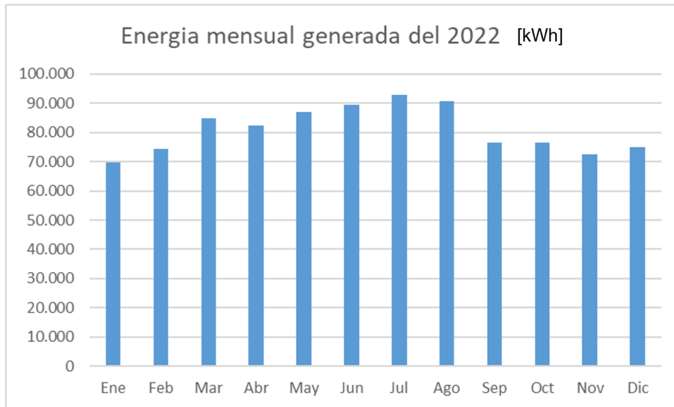
Figura 75 Energía mensual generada durante el año 2022 – Lago Posadas - SPSE
