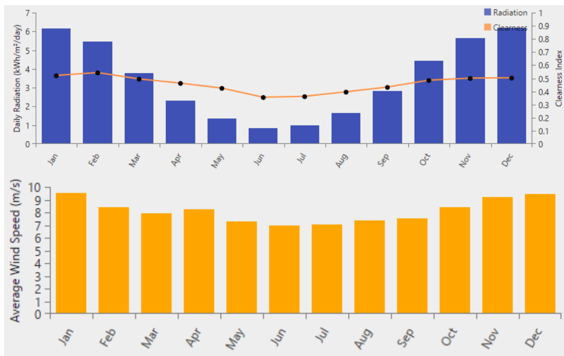
Figura 76 Recurso solar y eólico a la altura de simulación para Lago Posadas [HomerPro, 2023]
