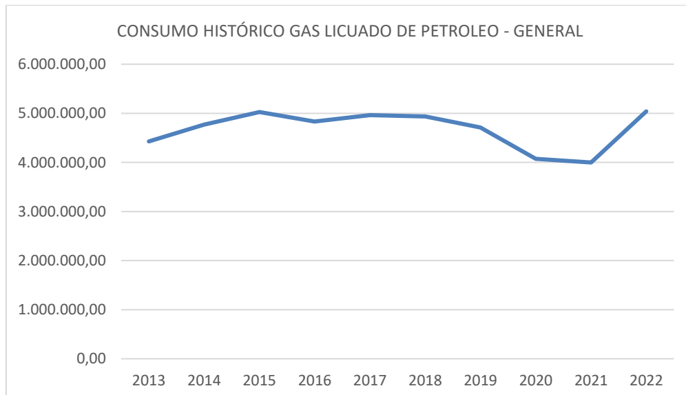
Figura 41 - Consumo histórico general de GLP [m 3 ] abastecido por Distrigas S.A. (Elab. Propia en
