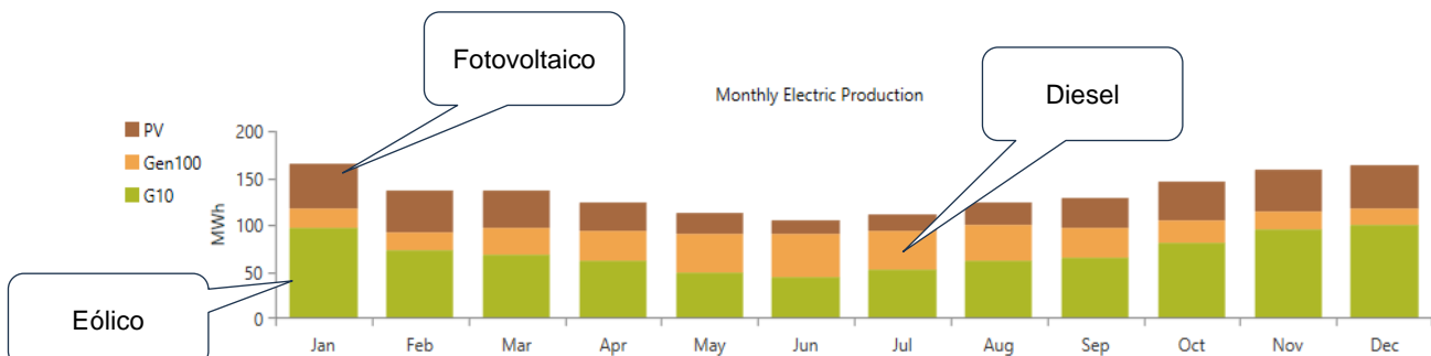
Figura 78 Resultados del escenario de simulación más favorable para Lago Posadas (elab.propia)
