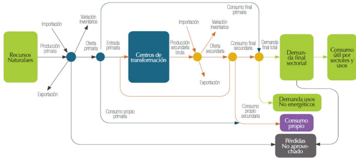
Figura 8 – Estructura del Balance Energético Nacional - Síntesis [DatosBE, 2022]
