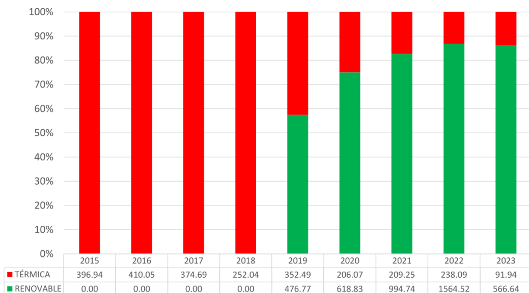
Figura 53 - Porcentajes de componente térmica (rojo) y renovable (verde) en la inyección de energía al SADI entre 2015 y 2022 para Santa Cruz, fuente [IESC-SPEME,2023]
