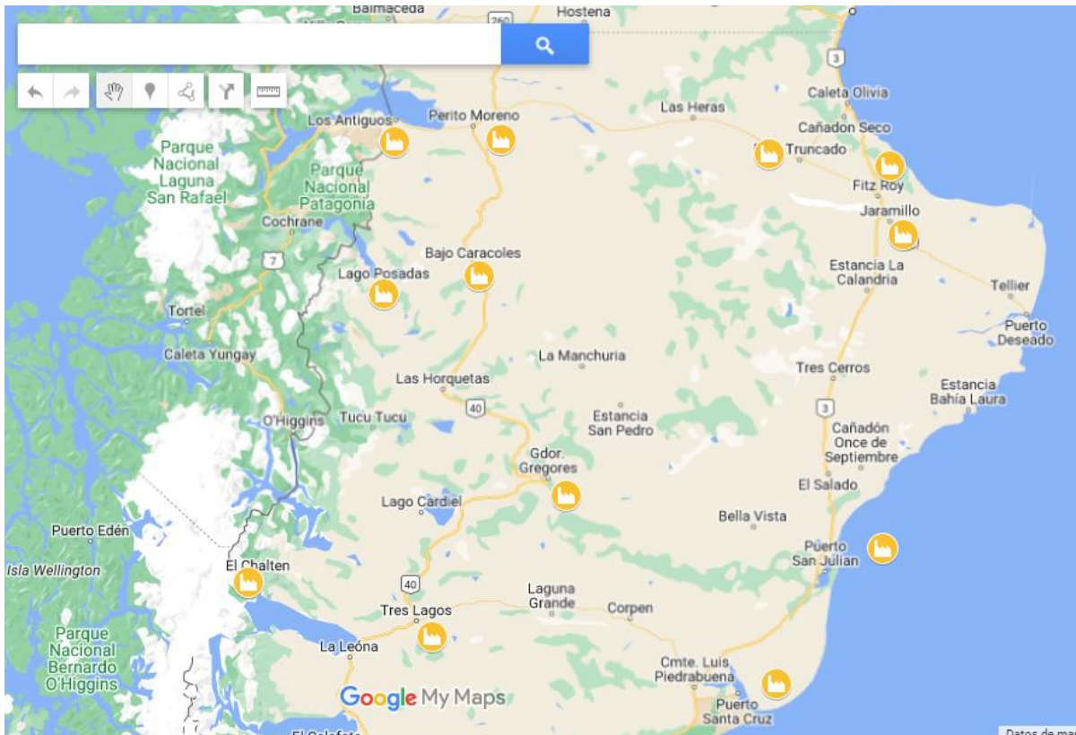
Figura 63 ubicación de centrales de generación aislada en zona norte y centro de Santa Cruz (elab.propia)
