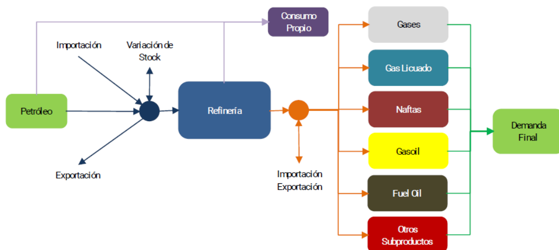
Figura 16 - Esquema de la cadena del petróleo según [MetodologíaBEN, 2015]
