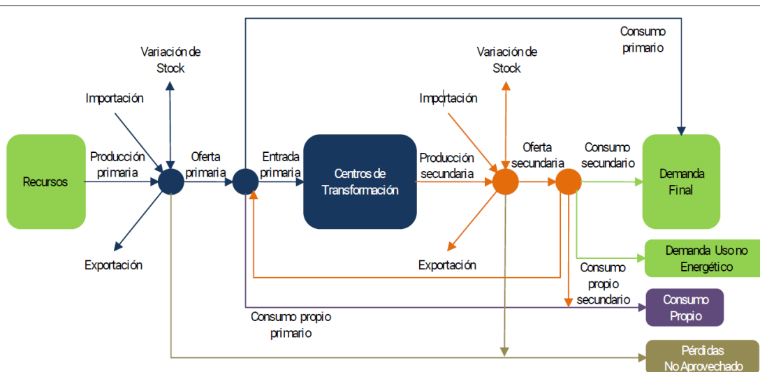
Figura 12 - Esquema de Oferta (Recursos), Transformación y Consumo en el BEN [MetodologíaBEN, 2015]
