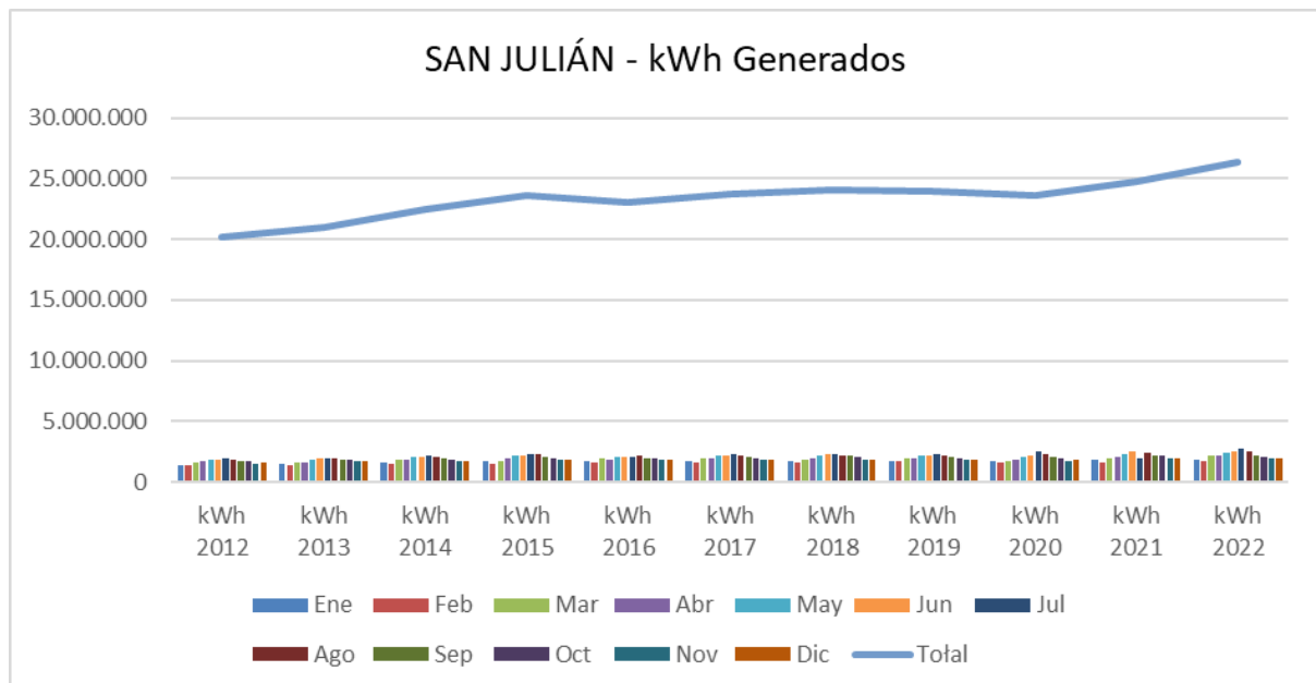
Figura 66 Datos de generación para la localidad de Puerto San Julián [SPSE-Mem421726,2023]
