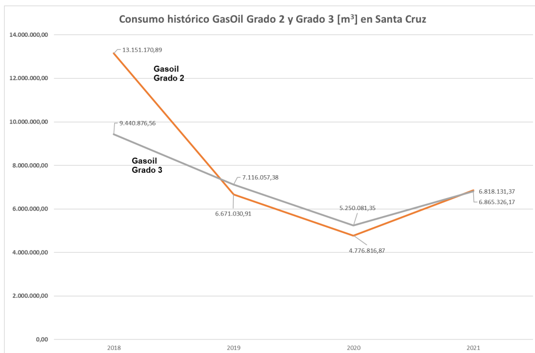
Figura 37 - Consumos históricos de Gas Oil Grado 2, Gas Oil Grado 3 en Santa Cruz 2018-2021 (Fuente: Elaboración Propia)
