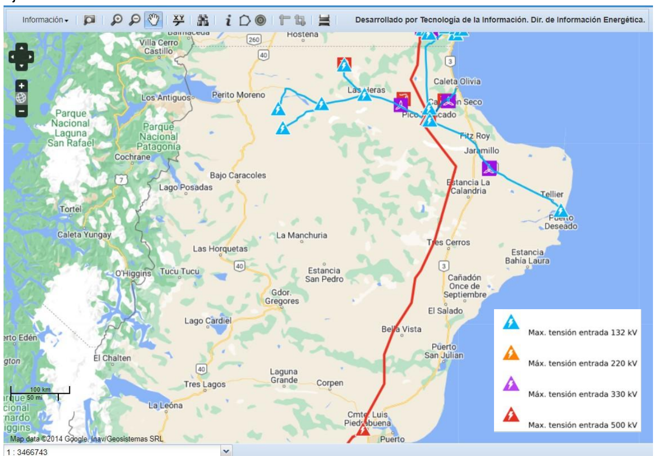
Figura 49 Vinculaciones al SADI en zona noreste de Santa Cruz [SIG-ENERGIA, 2023]
