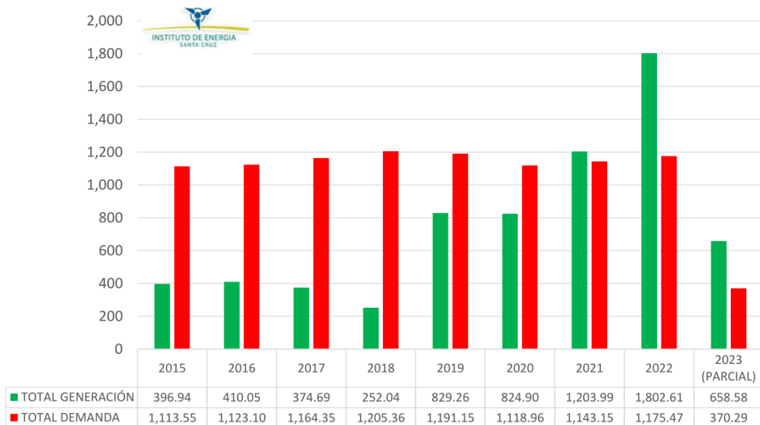
Figura 52 - Totales de generación y demanda anual [GWh] en Santa Cruz, con relación a intercambios en el SADI, fuente [IESC-SPEME,2023]
