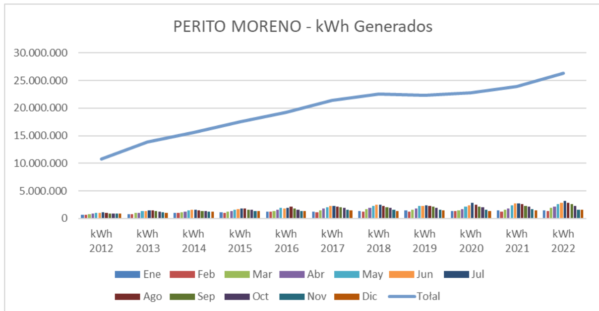
Figura 65 - Datos de generación para la localidad de Perito Moreno [SPSE-Mem421726,2023]
