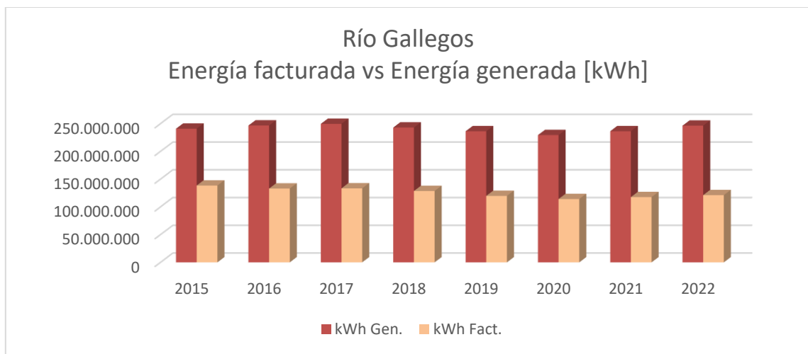
Figura 67 Comparativos entre energías facturada y generada / adquirida a SADI, para Río Gallegos (el.prop)
